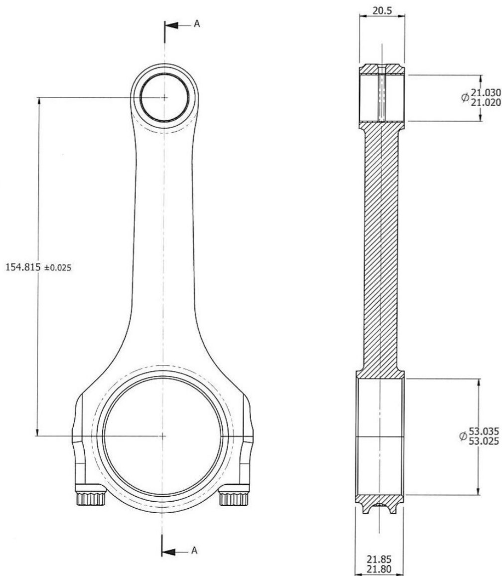
SECTION A-A
